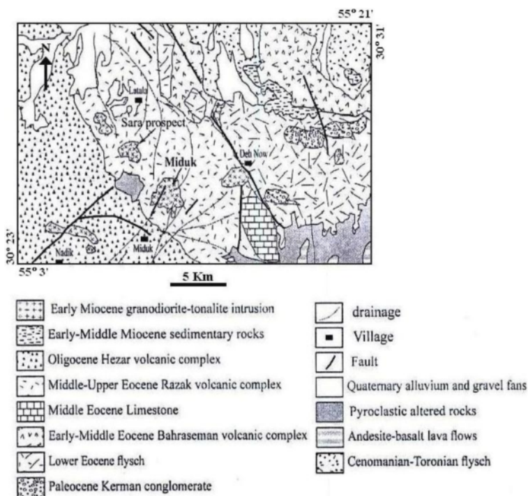
شکل ۲ نقشه زمین‌شناسی منطقه مورد بررسی - اقتباس با تغییرات از [۲۴].
