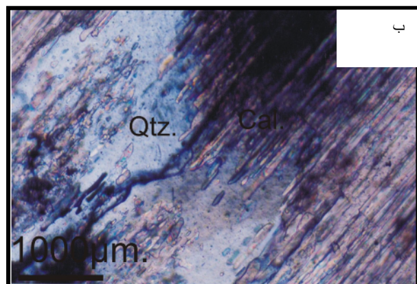
شکل ۱۴ الف تشکیل ژئپس و کلسیت در میانه و کوارتز در حاشیه رگچه، ب تشکیل کوارتزهای ثانویه بین کلسیت با بافت مرجانی (atoll texture) (نور قطبیده).
