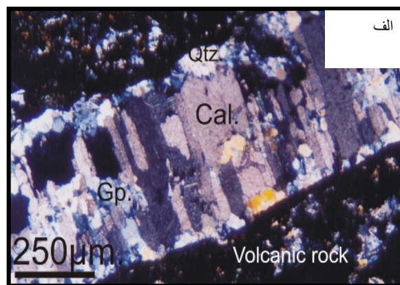
شکل ۱۴ الف تشکیل ژئپس و کلسیت در میانه و کوارتز در حاشیه رگچه، ب تشکیل کوارتزهای ثانویه بین کلسیت با بافت مرجانی (atoll texture) (نور قطبیده).
