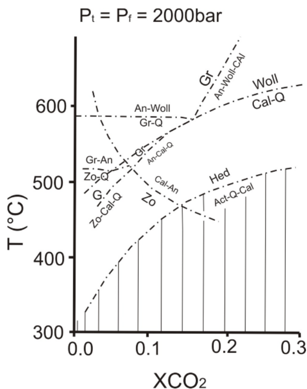
شکل ۶ با توجه به نمودار مقابل اکتینولیت در گستره دمائی (۳۲۰°C-۵۲۰°C) و در فشار کل ۲ کیلو بار پایدار است [۱۳].
