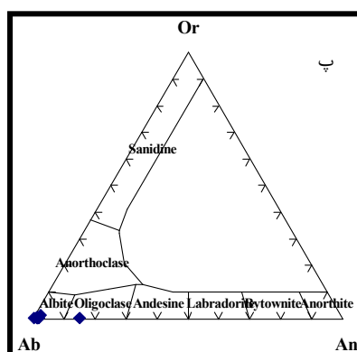
شکل ۹ الف. آلبیت‌های نوظهور در اثر دگرته‌ای نمک در سنگ‌های آتشفشانی گنبد نمکی دوآب تشکیل شده است، ب. تشکیل رگچه‌های کوارتز، کلسیت و آلبیت در سنگ‌های آتشفشانی گواه بر تاثیر دگرته‌ای در مراحل پایانی تبلور ماگماست (نور قطبیده)، پ. اغلب فلدسپات‌های مورد بررسی روی نمودار تقسیم‌بندی فلدسپات‌ها در گستره آلبیت قرار گرفته‌اند.
