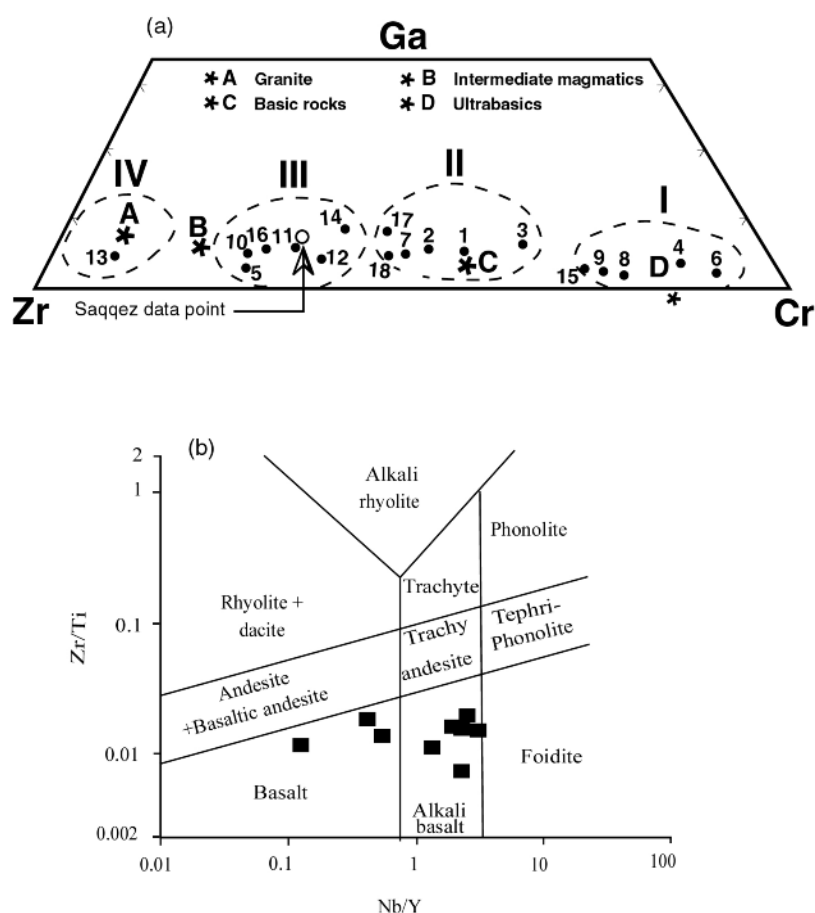
شکل ۸ (a) موقعیت نیمرخ دوم بوکسیتی سقز و مقایسه آن با کانسارهای بوکسیت کارستی و لاتریتی بر اساس مقادیر Zr , Cr و Ga آن‌ها. I, II, III و IV به ترتیب بیانگر مناطق اثر سنگ‌های مادر اولترامافیک، مافیک، حدواسط یا رسی، و اسیدی است. مقادیر متوسط Zr , Cr و Ga در سنگ‌های ماگمایی با حروف A, B, C و D نمایش داده شده‌اند که به ترتیب نشان دهنده محل قرارگیری سنگ‌های گرانیتی، سنگ‌های حدواسط، سنگ‌های آذرین بازیک و سنگ‌های اولترابازیک‌اند [۴۲]. شماره‌های ۱ تا ۱۸ به نهشته‌های بوکسیتی-لاتریتی مناطق مختلف جهان مربوط می‌شوند (به جدول ۳ مراجعه شود). (b) موقعیت کانسنگ‌های بوکسیتی سقز در دو متغیره Zr/Ti-Nb/Y [۴۷].
