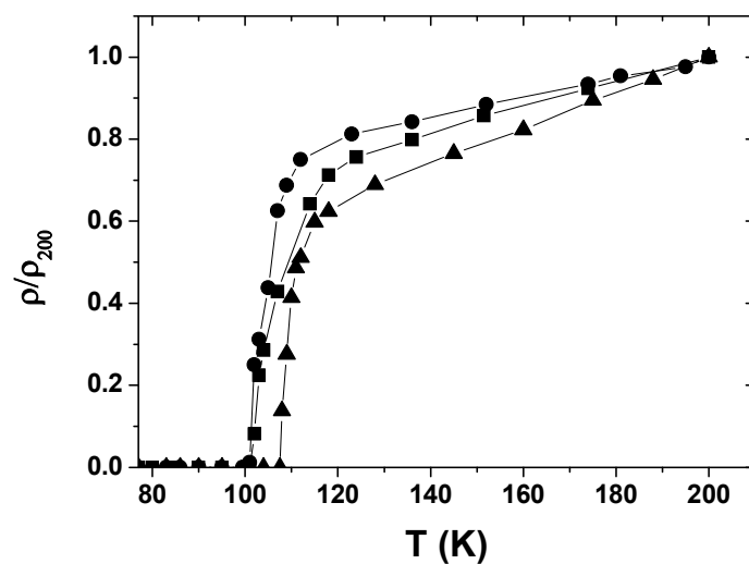
شکل ۵ نمودارهای \rho - T برحسب مقادیر متفاوت نانوذرات اکسید آنتیموان x = 0.07 (●) و x = 0.05 (▲) و x = 0.03 (■) با زمان پخت ۲۷۰ ساعت.
