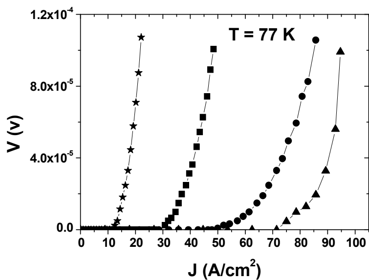
شکل ۹ نمودارهای V-I برای مقادیر متفاوت نانوذرات اکسید آنتیموان \text{Bi}_{0.7}\text{Sb}_{0.3} (★)، \text{Bi}_{0.5}\text{Sb}_{0.5} (▲)، \text{Bi}_{0.3}\text{Sb}_{0.7} (●)، \text{Bi}_{0.1}\text{Sb}_{0.9} (■) با زمان پخت ۲۷۰ ساعت.
