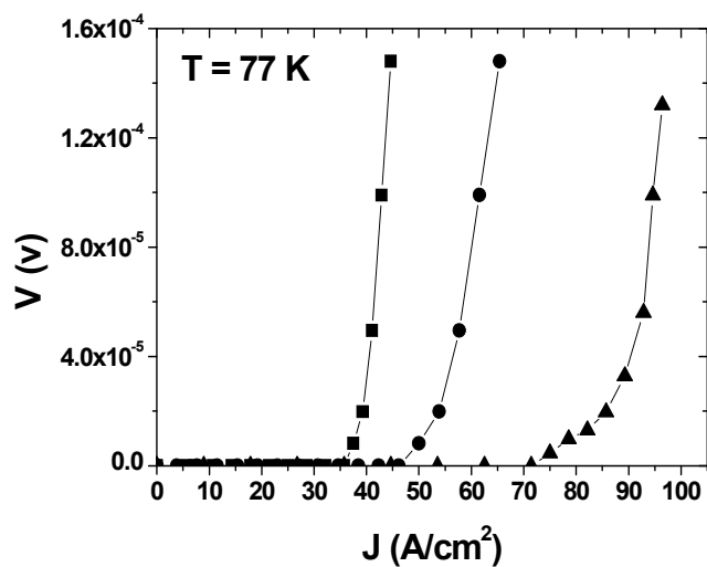
شکل ۱۰ نمودارهای V-I با زمان‌های پخت ۱۵۰ (■)، ۲۱۰ (●)، ۲۷۰ (▲) ساعت برای نمونه‌ای با مقدار نانوذرات اکسید آنتیموان \text{Bi}_{0.5}\text{Sb}_{0.5} x = 0.5 .
