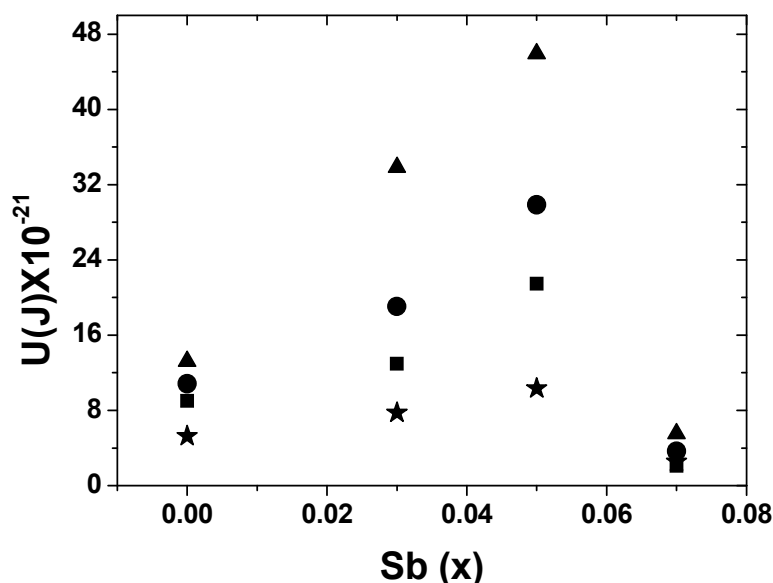
شکل ۱۶ انرژی فعال‌سازی بر حسب مقادیر نانوذرات اکسید آنتیموان در ابررسانای پایه‌ی بیسموت با زمان‌های پخت ۱۵۰ (★)، ۲۱۰ (●)، ۲۷۰ (▲) و ۳۳۰ (■) ساعت.
