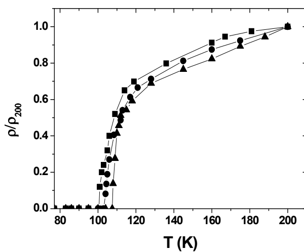
شکل ۶ نمودارهای \rho - T برای زمان‌های پخت ۲۱۰ (●)، ۱۵۰ (■)، و ۲۷۰ (▲) ساعت نمونه‌ای با مقدار نانوذرات اکسید آنتیموان x = 0.05 .
