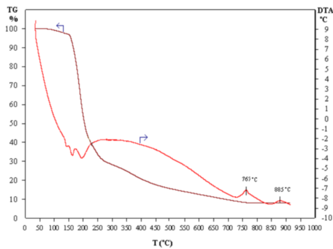
شکل ۳ منحنی TG و DTA ژل خشکیده ی YIG.
