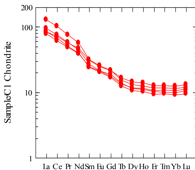
شکل ۶ نمودار عناصر خاکی در سنگ‌های مورد بررسی که نسبت به کندریت [۲۰] بهنجار شده اند. غنی‌شدگی از عناصر نادر خاکی سبک (LREE) و تهی‌شدگی از عناصر نادر خاکی سنگین (HREE) را نشان می‌دهند.
