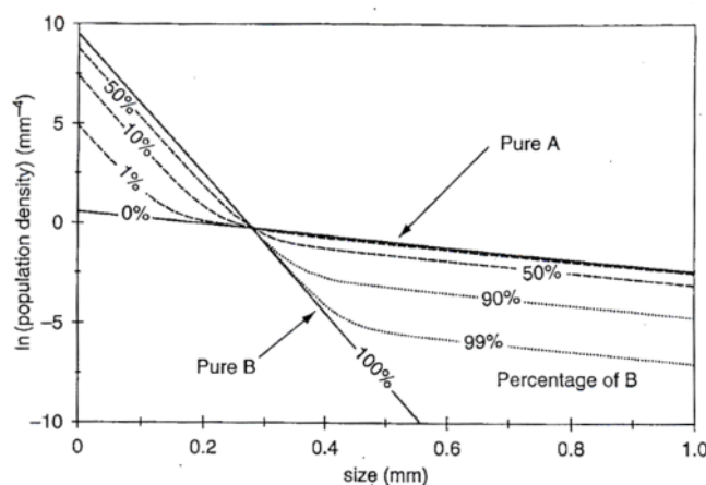
شکل ۳ اضافه شدن دو CSD خطی به یکدیگر و ایجاد CSD منحنی وار. شیب‌های اولیه دو تشکیل دهنده‌ی CSD برای اندازه‌های بزرگ و کوچک حفظ می‌شود ولی عرض از مبدا آن‌ها حفظ نمی‌شود.
