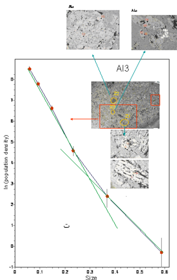
ادامه شکل ۸ (ت) چگونگی خمش در نمودارهای وابسته به CSD در فنوکریست‌های آمفیبول مورد بررسی (مقاطع نازک متعدد مورد بررسی با بلورهای آمفیبول بزرگ و کوچک).
