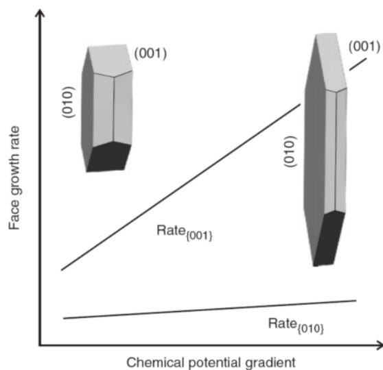
شکل ۸ واکنش احتمالی سرعت‌های رشد وجوه پلاژیوکلاز به تغییرات گرادیان پتانسیل شیمیایی پیرامون بلور در حال رشد [۲۰]. سطح (۰۰۱) به‌عنوان سطح حاشیه‌ی تخته انتخاب شده است (فرض بر این است که سرعت رشد سطوح (۱۱۰)، (۱۰۱) و (۱۱۰) معادل با سطح (۰۰۱) است). اندازه‌ی کلی بلور نمایش داده شده سرعت رشد و زمان تبلور را بازتاب می‌دهد.
