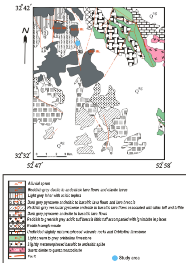
شکل ۳ نقشه‌ی زمین‌شناسی ساده شده‌ی منطقه (برگرفته از [۲۰] با تغییرات).
