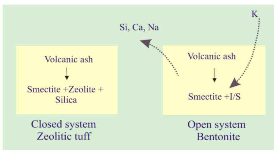
شکل ۱. مقایسه‌ی تبدیل مواد آتشفشانی شیشه‌ای اسیدی به توف زئولیتی در یک سیستم بسته و به اسمکتیت (بنتونیت) یا کانی‌های ایلیت-اسمکتیت در یک سیستم باز که عناصر شیمیایی به سیستم وارد و یا خارج می‌شوند (برگرفته از [۱۵]).
