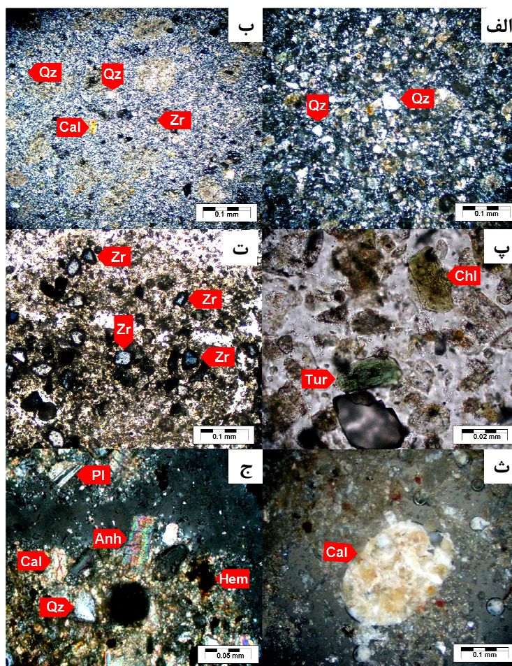
شکل ۲ (الف): فراوانی کوارتزهای درشت دانه (Qz) در حد ماسه خیلی ریز دانه تا سیلت درشت دانه (۰/۱۲۵-۰/۰۳۱ میلی‌متر) در مقاطع شمال شرقی (XPL)؛ (ب): کاهش اندازه ی ذرات تشکیل دهنده بادرفت‌ها در حد سیلت میان دانه تا رس (۰/۰۳۹-۰/۰۱۵۶ میلی‌متر) در مقاطع جنوب غربی (کوارتز (Qz) + زیرکن (Zr) + کربنات کلسیم (Cal) (XPL)؛ (پ): درشت بلور تورمالین (Tur) + کلریت منیزیم دار (Chl) (PPL)؛ (ث): زیرکن‌های درشت دانه (Zr) با حاشیه متامیکتی در مقاطع شمال شرق (PPL)؛ (ج): کربنات کلسیم (Cal) با بافت هسته ریخت (Cytomorphic) (XPL) و (ج): انیدریت (Anh) + پلاژیوکلاز (Pl) + هماتیت (Hem) + کربنات کلسیم (Cal) (XPL).
