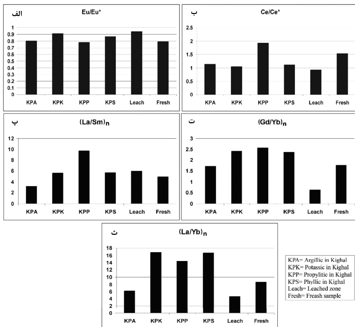
شکل ۳ نمودارهای ستونی مقادیر متوسط (\text{Eu}/\text{Eu}^*) ، (\text{Ce}/\text{Ce}^*) ، (\text{La}/\text{Yb})_n و (\text{La}/\text{Sm})_n برای زون‌های مختلف دگرسان، بهنجار شده نسبت به کندریت [۱۸].
