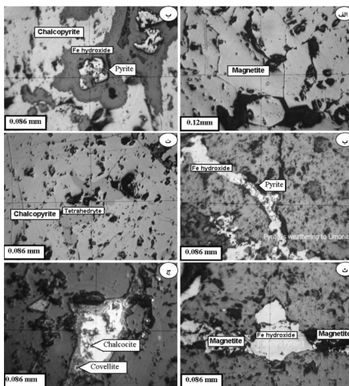
شکل ۷ (الف) دانه های خود شکل مگنتیت با بافت موزائیکی (ب) پیریت خود شکل که با کالکوپیریت احاطه شده است (پ) شکل گیری پیریت به صورت رگچه ای و پدیده ی جانشینی پیریت به وسیله ی لیمونیت (ت) اداخل کانی چهاروجهی در کانی کالکوپیریت (ث) تبدیل پیریت و مگنتیت به هیدروکسیدهای آهن (ج) جانشینی کانی کوولیت در حاشیه ی کانی کالکوسیت.
