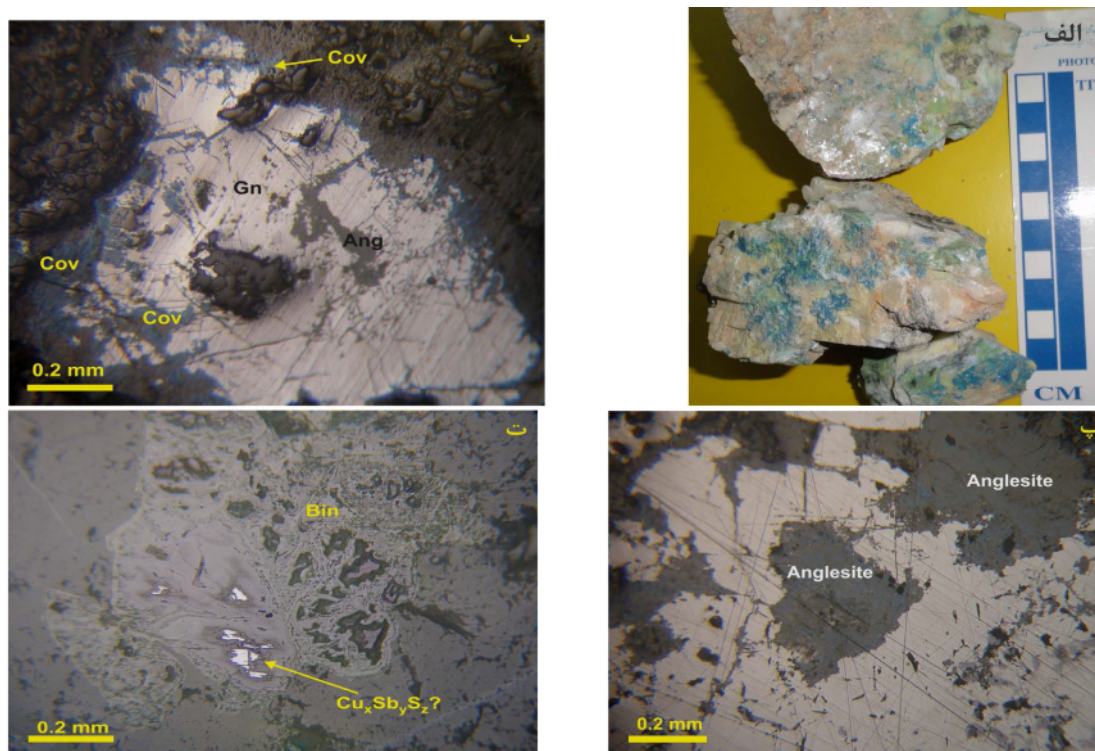
شکل ۷ تصاویری از کانی‌سازی ثانویه زون اکسایشی الف) مالاکیت و آزوریت همراه با باریت (نمونه‌ی Si-44)، ب) کوولیت همراه با آنگلیزیت در حاشیه‌ی گالن (نمونه‌ی Si-43 نور PPL)، پ) آنگلیزیت همراه با کوولیت در اطراف گالن (نمونه Si-50 نور PPL)، ت) تبدیل سولفید مس-آنتیموان به کانی بیندهمیت با بافت کلوفر (نمونه Si-44 نور PPL). Gn = گالن، Cov = کوولیت، Ang = آنگلیزیت، Bin = بیندهمیت
