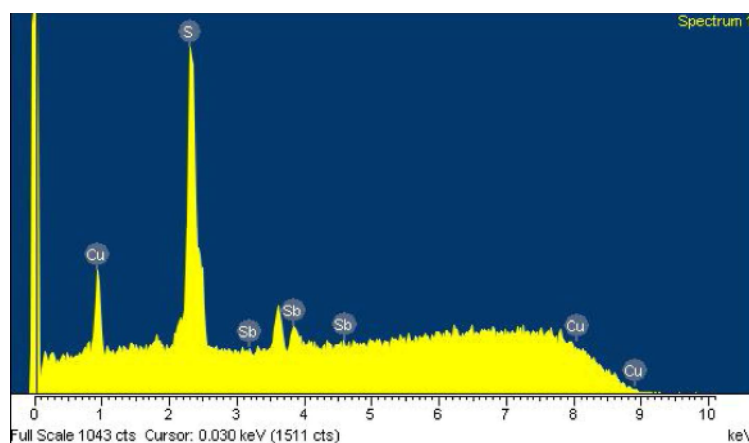
شکل ۱۱ تجزیه‌ی عنصری کانی ناشناخته در نمونه Si-44 با SEM.
