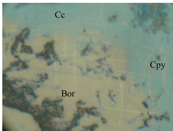
شکل ۱۲ جدایش کالکوپیریت در بورنیت. در اثر هوازدگی بورنیت به کالکوسیت تبدیل شده ولی تیغه‌های کالکوپیریت سالم مانده است.
