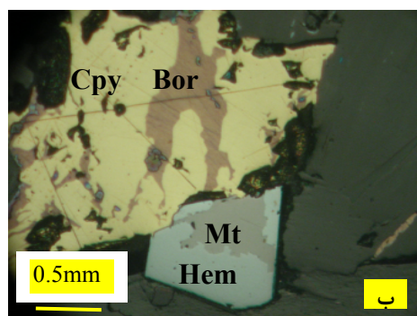
شکل ۱۱ الف) رگچه‌های تیره رنگ مگنتیت، بیوتیت و آمفیبول همراه با کانی‌سازی مس در شمال صفی خانلو. ب و پ) همراهی اکسیدهای آهن با کانی‌های سولفیدی مس در کانی‌سازی رگچه‌ای.
