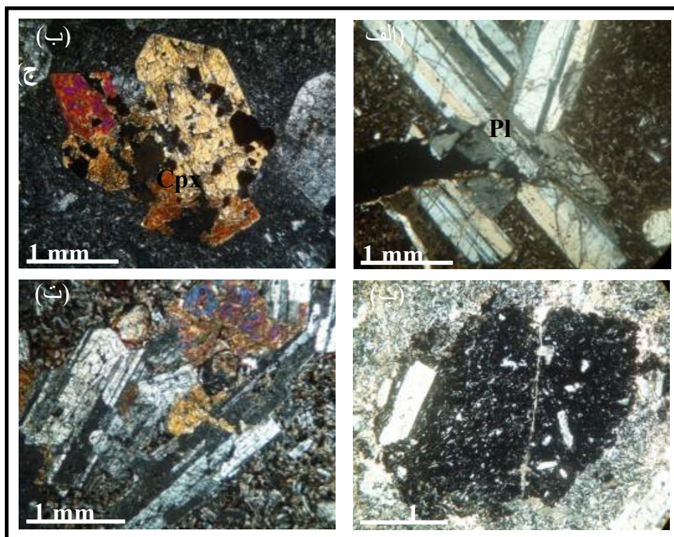
شکل ۴ تصاویر میکروسکوپی از (الف): فنوکریست پلاژیوکلاز با بافت غربالی و گلومروپورفیری و (ب): فنوکریست پیروکسن وابسته به سنگ‌های آندزیتی (وضعیت XPL)، پ و ت برونوم‌های ماگمایی ریزدانه و درشت دانه در گدازه‌های منطقه مورد بررسی (وضعیت XPL).
