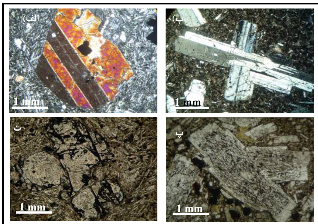
شکل ۳ تصاویر میکروسکوپی از (الف): فنوکریست پیروکسن با ماکل پلی سنتتیک (XPL) (ب): فنوکریست‌های پلاژیوکلاز (XPL) (پ): بلورهای ایدنگزیتی شده البوین وابسته به سنگ‌های بازالتی، (PPL) (ت) فنوکریست‌های پلاژیوکلاز با بافت غربالی و نامتعادلی در سنگ‌های آندزیت بازالتی، (PPL).
