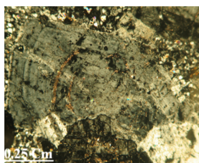
شکل ۵ تصاویری از فنوکریست‌های پلاژیوکلاز (Pl) وابسته به توده‌ی نفوذی میدوک پورفیری ک ماکل‌های پلی‌سنتتیک و منطقه‌بندی نوسانی در آن‌ها دیده می‌شود و نیز تحت تأثیر دگرسانی تا حدودی سریسیتی و کلریتی شده‌اند- نور XPL.
