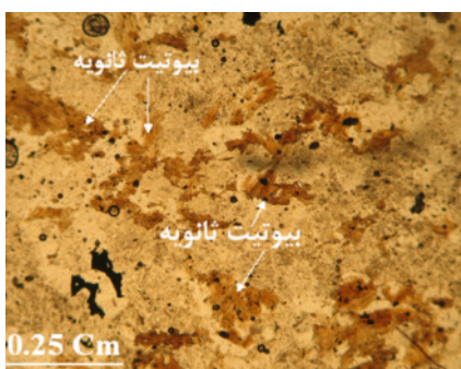
شکل ۷ انواع بیوتیت‌های موجود در توده گرایتوئیدی میدوک پورفیری (شکل سمت راست نور XPL و شکل سمت چپ نور PPL).
