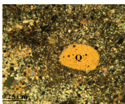
شکل ۶ فنوکریست‌های کوارتز با حواشی انحلالی و خلیجی- نور XPL.
