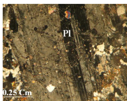
شکل ۵ تصاویری از فنوکریست‌های پلاژیوکلاز (Pl) وابسته به توده‌ی نفوذی میدوک پورفیری ک ماکل‌های پلی‌سنتتیک و منطقه‌بندی نوسانی در آن‌ها دیده می‌شود و نیز تحت تأثیر دگرسانی تا حدودی سریسیتی و کلریتی شده‌اند- نور XPL.
