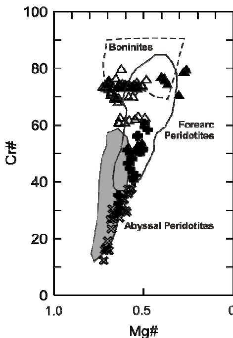
شکل ۶ الف) نمودار Mg\# نسبت به Cr\# برای کروم اسپینل‌های مختلف واحدهای مختلف مجموعه ده شیخ، محدوده آبیسال پریدوتیت‌ها به نقل از دیک و بولن [۶] و آرای [۷] و گستره‌ی پریدوتیت‌های جلوی قوس به نقل از بلومر و هاوکینس [۱۷]، بلومر و فیشر [۱۸]، ایشی و همکاران [۱۹] و پارکینسون و پیرس [۲۰] و گستره‌ی بونینیت‌ها از یومینو [۲۱]، وان در وال [۲۲]، کامرون [۲۳]، سوبولو و دانیوشوسکی [۲۴] می‌باشد.
