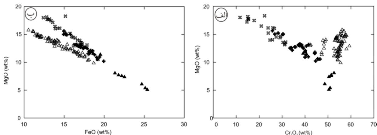
شکل ۵ الف و ب- تغییرات ترکیبی اسپینل در واحدهای مختلف سنگ‌شناسی مجموعه ده شیخ از جمله هارزبورژیت‌ها، لِرزولیت‌ها، دونیت‌ها و کرومیت‌ها.
