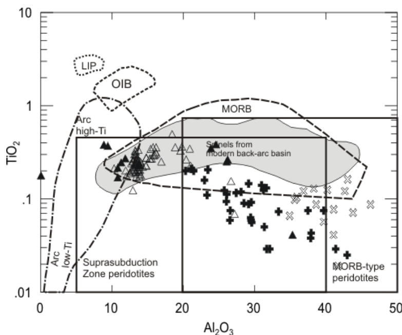
شکل ۷ تغییرات TiO_2 (wt%) نسبت به Al_2O_3 (wt%) در کروم اسپینل‌های موجود در سنگ‌های مختلف مجموعه ده شیخ و موقعیت آن‌ها نسبت به محیط‌های زمین‌ساختی مختلف. گستره‌های زمین‌ساختی مختلف به نقل از کامنستکی و همکاران [۳۳] است. چنانکه مشاهده می‌شود کرومیت‌های ده شیخ در گستره‌ی کروم اسپینل‌های وابسته به چند فرورانشی قرار می‌گیرند.
