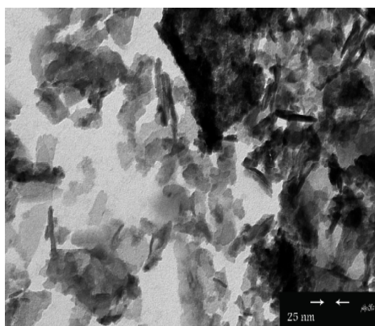
شکل ۲ تصاویر TEM وابسته به نانوذرات نمونه (a).
