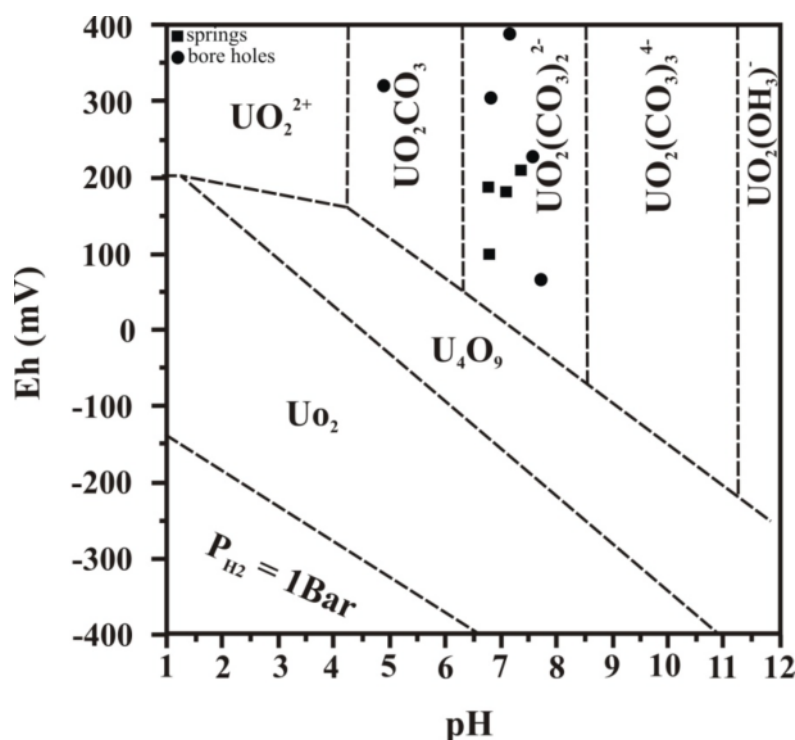
شکل ۶ نمودار Eh/pH گونه‌های محلول در آب و فازهای جامد سیستم U-O 2 -C-H 2 O در دمای (°C) ۲۵ و [۵] U = 1.3 \times 10^{-4} M, C = 2.3 \times 10^{-3} M.
