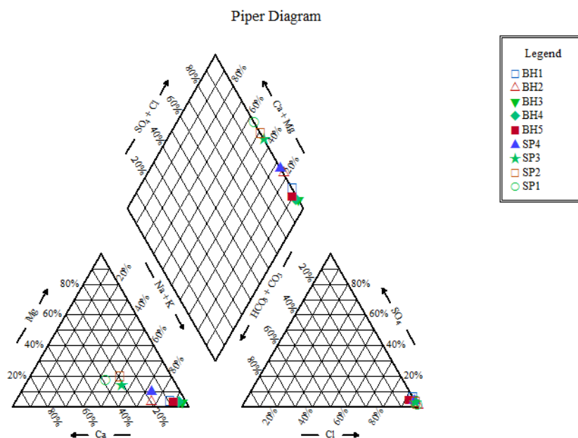
شکل ۳ نمودار پای پر نمونه‌های آب گمانه‌های منطقه آیرکان و چشمه‌های منطقه چشمه شتری..
