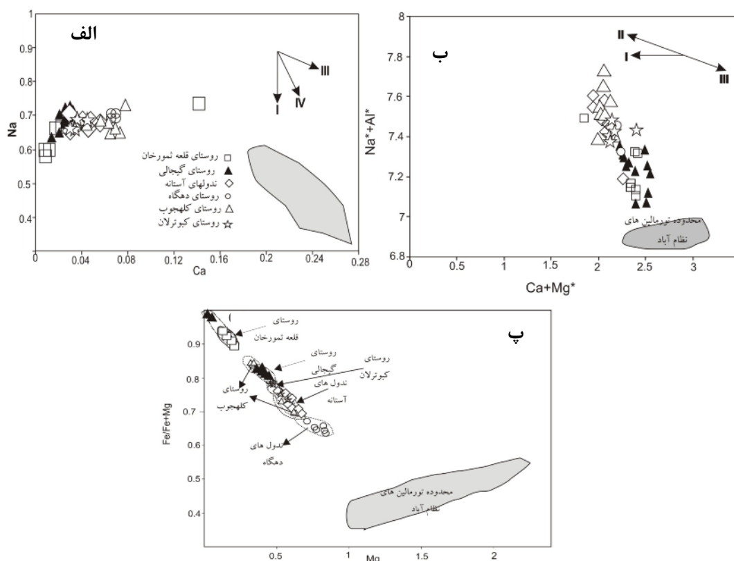
شکل ۴ الف: ترسیم نمونه‌ها در نمودار Ca نسبت به Na. ب: همبستگی وارون Ca + Mg^* نسبت به Na^* + Al . Mg^* = Mg + Fe + Mn + Na^* + Al . ج: همبستگی وارون Fe/Fe + Mg نسبت به Mg . نمودار ۲: 2Li - Ti , Na^* = Na + K , Al^* = Al + Fe^{3+} + 2Ti - Lic . تورمالین‌های دهگاه و بالاتر بودن میزان Fe/Fe + Mg در نمونه‌های رگه‌های روستای کبوتران و گيجالی است.
