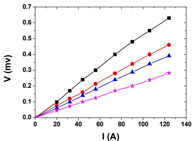
شکل ۶ نمودار V-I برای نمونه‌های آلایش داده شده در دمای اتاق با مقادیر مختلف نانوذرات طلا (■) ۰/۰٪، (●) ۰/۵٪، (▲) ۱٪ و (★) ۲٪ با زمان پخت ۷۲ ساعت.
