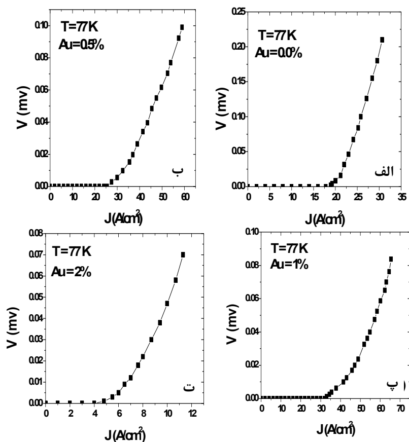
شکل ۵ نمودارهای V-I برای مقادیر متفاوت نانوذرات طلا (الف، ۰/۰٪، ب، ۰/۵٪، ج، ۱٪ و د، ۲٪) با زمان پخت ۷۲ ساعت.
