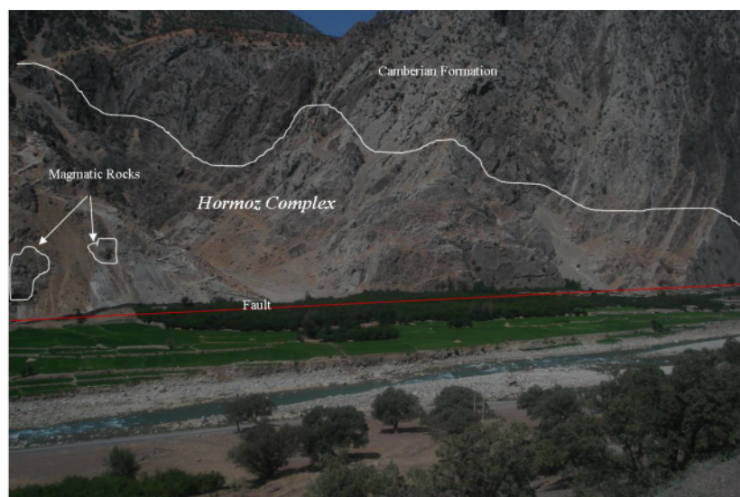
شکل ۳ رخنمون مجموعه سازندهای تبحیری (گنبد نمکی) در امتداد گسل‌ها.
