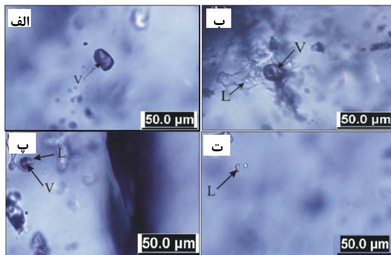
شکل ۸ الف) شاره‌ی درگیر تک فاز گاز (V)، ب) شاره‌ی درگیر دو فاز (L) فاز مایع و (V) فاز گاز، پ) شاره‌ی درگیر تک فاز آبگون (L)، ت) شاره‌ی درگیر دو فاز (L) فاز گاز و (L) فاز آبگون.
