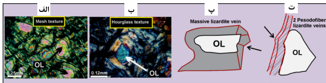
شکل ۴ - الف- بافت شبکه‌ای در سنگ مادر هارزبورژی (در نور تداخلی). ب- بافت ساعت شنی در سنگ مادر دونیتی با هسته الیوینی که هنوز به سرپانتین تبدیل نشده است (در نور متقاطع). پ- تصویر نموداری از چگونگی رشد رگه لیزاردیت توده‌ای در محل فرورفتگی دانه الیوین. ت- تصویر نموداری از چگونگی رشد رگه شبه فیبری لیزاردیت در محل برجستگی الیوین.
