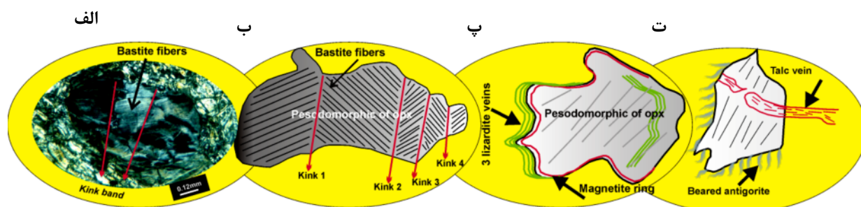
شکل ۹ الف- ارتوپروکسن باستیتی شبه ریخت که هنوز شکنج اولیه ارتوپروکسن در آن قابل تشخیص است (در نور متقاطع). ب- تصویر نموداری از چهار نوار شکنجی در یک ارتوپروکسن اولیه که رشته‌های باستیت ثانوی در جهت انحنا شکنجهای اولیه رشد کرده، ضمن این که خاموشی موجی را نیز حفظ کرده‌اند. پ- تصویر نموداری از تشکیل حلقه مگنتیتی در پیرامون ارتوپروکسن شبه ریخت و حفظ شکل اولیه ارتوپروکسن. رگه‌های لیزاردیتی بعدی نیز از همین الگو پیروی کرده‌اند. ت- رشد آنتی‌گوریت‌های ریشه‌مانند در اطراف ارتوپروکسن باستیتی شده و حفظ شکل اولیه آن.
