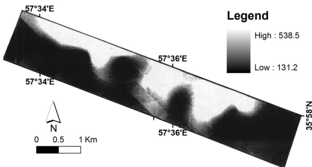
شکل ۱۱ مولفه‌ی اصلی شماره سه عناصر تجزیه شده در نمونه‌های سنگی. مناطق روشنتر همراهی عناصر Cu, Zn, F, Sr را نشان می‌دهند.
