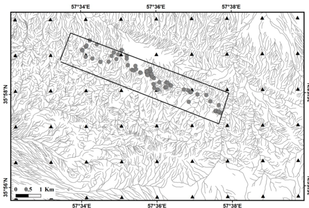
شکل ۳ موقعیت نمونه‌های ژئوشیمیایی رسوب آبراهه‌ای (نقاط ● از [۲۰، ۱۹، ۱۳، ۲۱] و ▲ از [۱۸] استخراج شده است).
