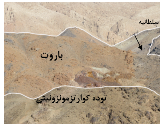
ب- تزریق توده در سازند باروت و ایجاد کانه‌زایی آهن و منگنز در آن.
