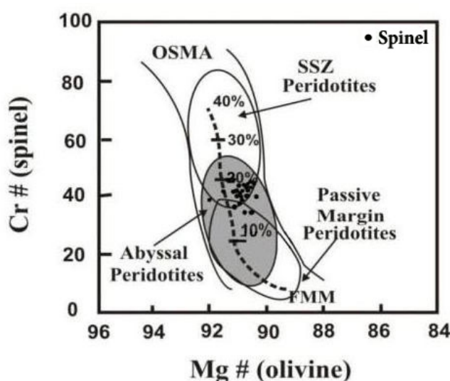
شکل ۷ الف: نمودار Al_2O_3 نسبت به Cr_2O_3 در اسپینل که خاستگاه گوشته ای اسپینل ها را نشان می دهد. [۲۳، ۲۲، ۲۱]. ب- Cr^\# اسپینل نسبت به Mg^\# الیوین های همزیست در پریدوتیت که نشان دهنده ترکیب OSMAs و abyssal است. [۲۴].
