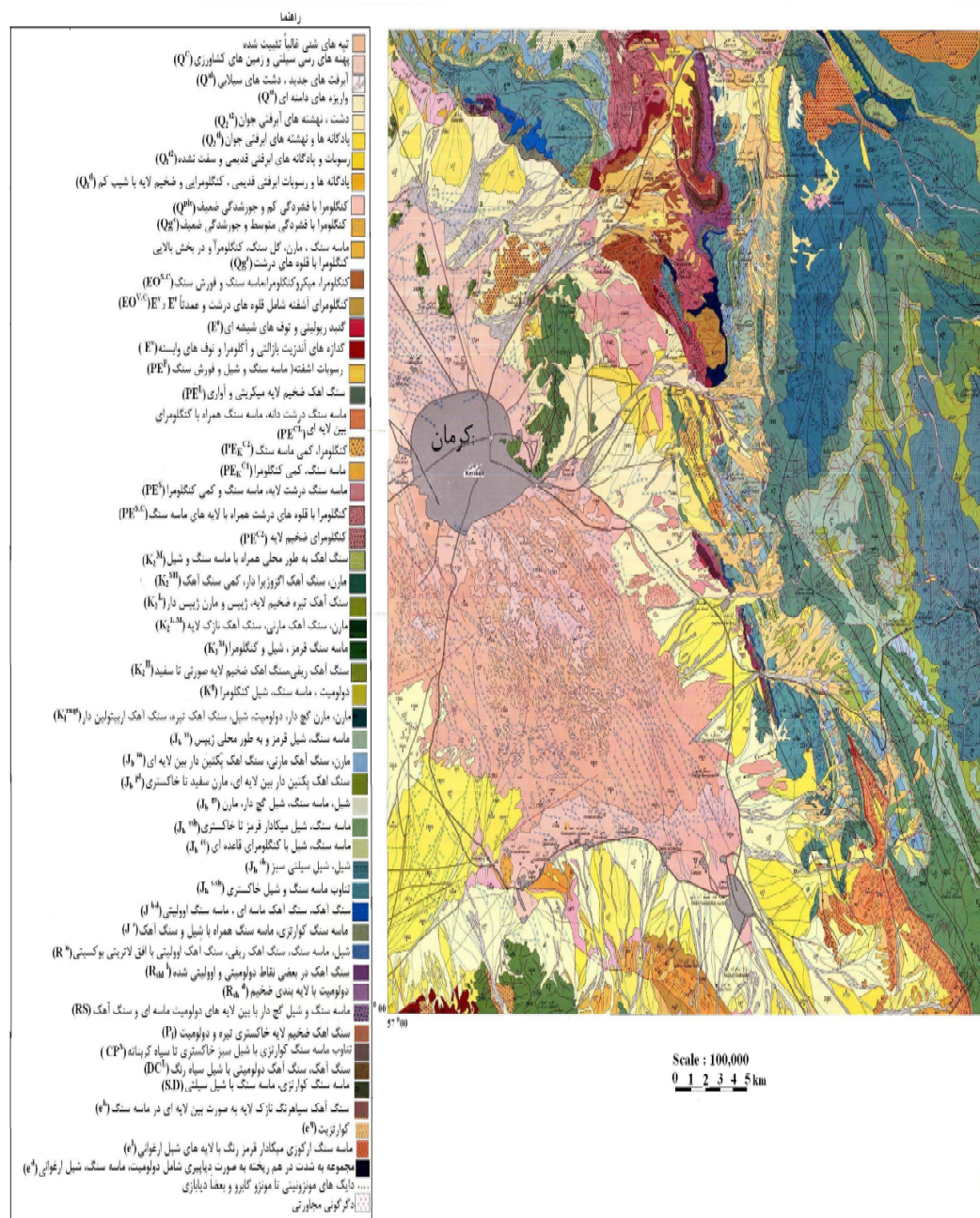
شکل ۳ نقشه ی زمین شناسی شهر کرمان و حومه.
