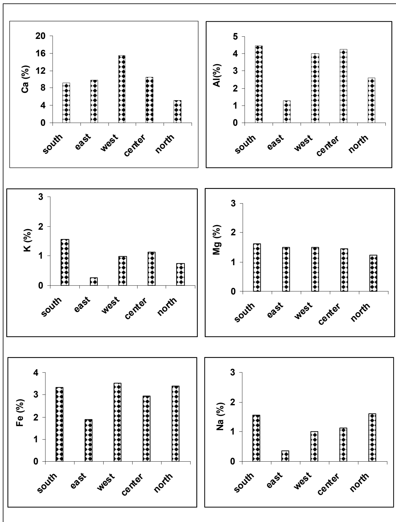
شکل ۱۴ تغییرات غلظت عناصر K, Na, Mg, Al, Fe و Ca در غبار مناطق مختلف شهر کرمان.
