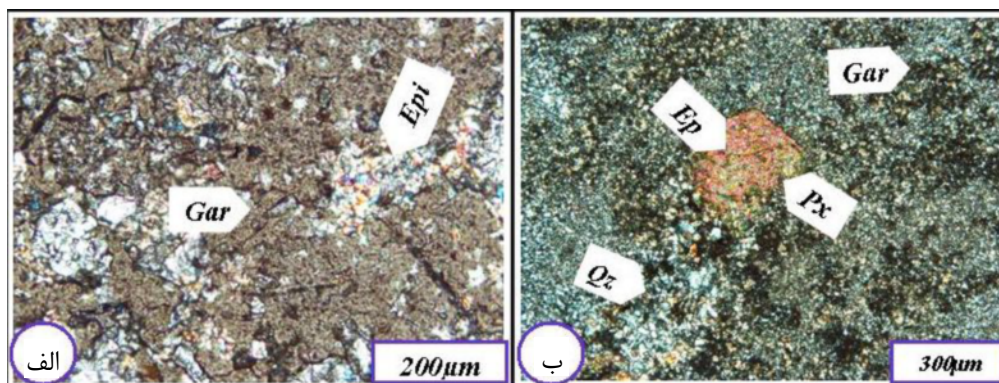
شکل ۳ الف) گارنت‌های زون اسکارن درونی که با توجه به ویژگی‌های نوری از نوع گرانادیت‌اند (XPL) ب) قالبی از کانی پیروکسن که با کانی اپیدوت در زون اسکارن بیرونی پر شده است (XPL).
