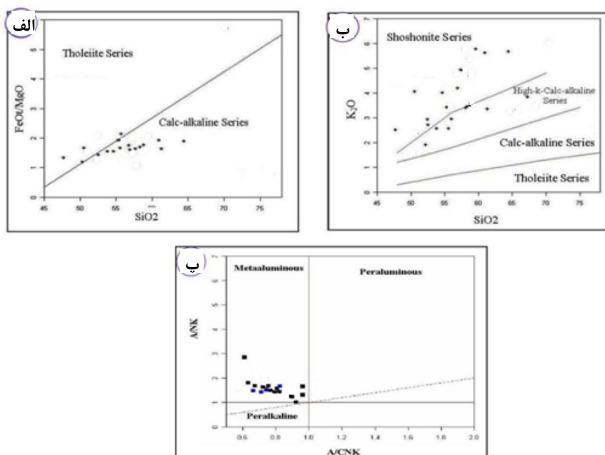
شکل ۵ (الف) موقعیت نمونه‌های توده‌ی نفوذی در نمودار \text{FeO/MgO-SiO}_2 [۸] (ب) نمودار \text{SiO}_2 نسبت به \text{K}_2\text{O} [۹] (پ) نمودار \text{A/NK} [۱۰].
