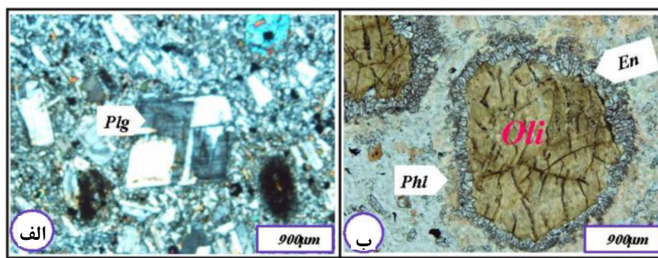
ب) دگرسانی الیوین به انستاتیت و فلوگوپیت (XPL).
