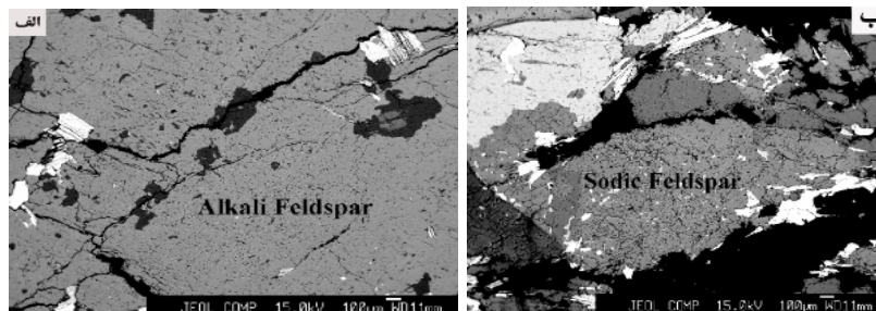
ی. میکروسکوپ الکترونی (BSE) فلدسپارهایی از منطقه ی سنگین آباد . الف) فلدسپارهای قلیایی سرشار از ارتوکلاز ؛ ب) آلبیت.
