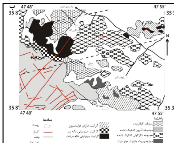
۱ ساختاری ایران (اقتباس از [۱۰]). موقعیت منطقه‌ی مورد بررسی با مربع سیاه رنگ مشخص شده است. (ب) نقشه‌ی زمین-پاس ۱:۱۰۰۰۰۰ بر پایه‌ی [۱۵].
