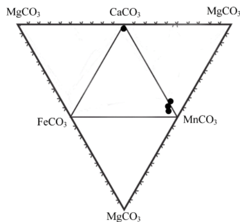
شکل ۹ ترکیب ۴ نمونه از کربنات موجود در زیر واحد توف‌آهکی ( E_6^{vct} ) در نمودار چهار سازندی (سیستم) کلسیت - رودوکروزیت - منیزیت - سیدریت. دایره‌های توپر نشان‌دهنده‌ی ترکیب کربنات‌های کانسار بزنین هستند. سیدریت: (FeCO_3) ؛ رودوکروزیت: (MnCO_3) ؛ کلسیت: (CaCO_3) و منیزیت: (MgCO_3) .
