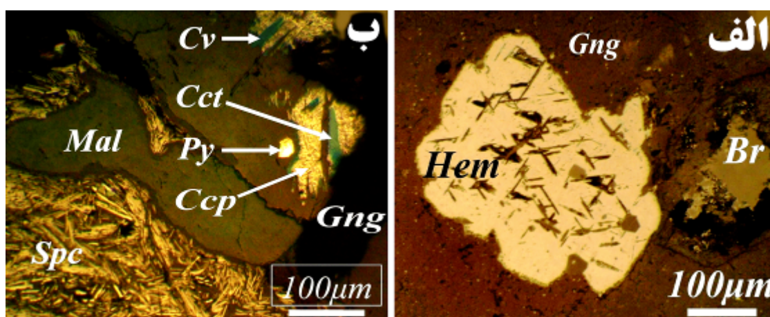
شکل ۶ (الف) هماتیت (Hem) جانشین مگنتیت شده و رخ‌های مگنتیت به صورت روشنی حفظ شده‌اند. در سمت راست مگنتیت اکسید شده، براونیت (Br) در زمینه‌ی باطله‌ی کربناتی - سیلیکاتی (Gng) مشاهده می‌شود. نور بازتابی طبیعی. (ب) کانی‌های سولفید مس کالکوسیت (Cct)، کوولیت (Cv) و کالکوپیریت (Ccp) به همراه پیریت (Py) در زمینه‌ی مالاکیت (Mal) و در اطراف مالاکیت، بلورهای سوزنی و کشیده اسپیکولاریت (Spc) دیده می‌شوند. نور بازتابی طبیعی.
