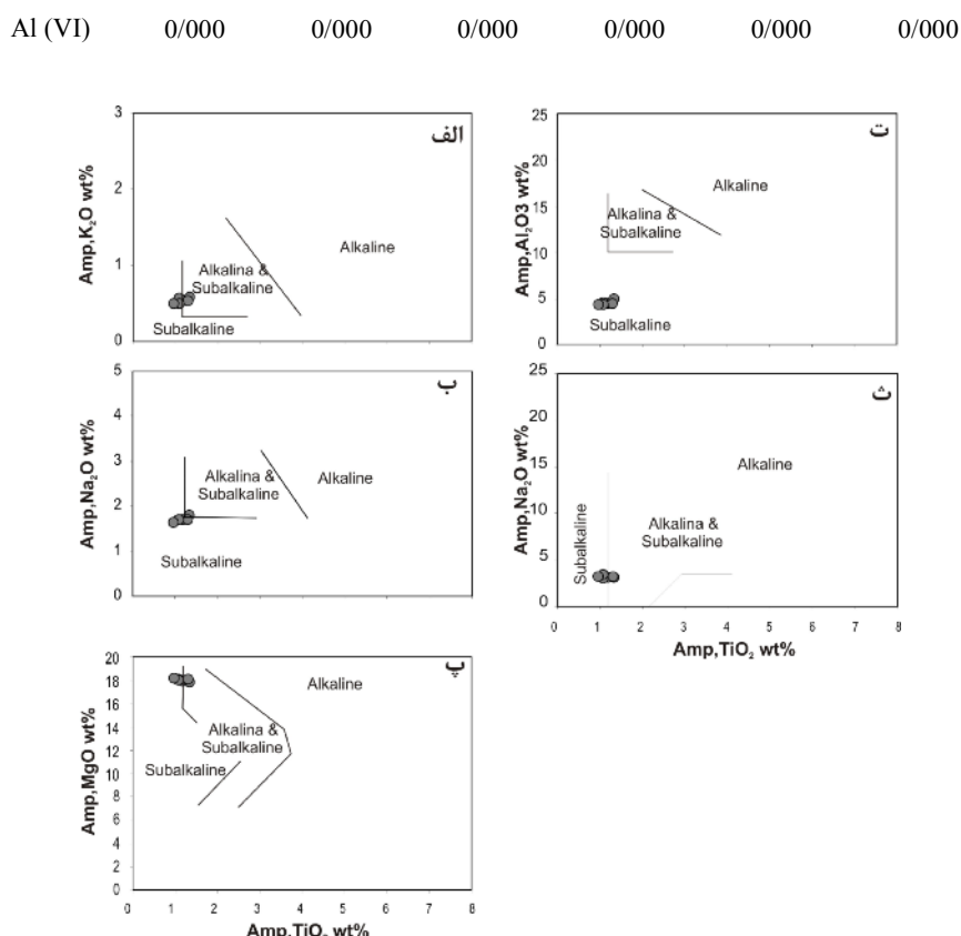
شکل ۱۴ در نمودارهای \text{TiO}_2 (نسبت به الف) \text{K}_2\text{O} ، ب) \text{Na}_2\text{O} ، پ) \text{MgO} ، ت) \text{Al}_2\text{O}_3 ، و ث) \text{Na}_2\text{O}/\text{K}_2\text{O} حاصل از آنالیز آمفیبول‌ها ماهیت ماگما به نیمه‌قلیایی تمایل دارد [۳۴].
