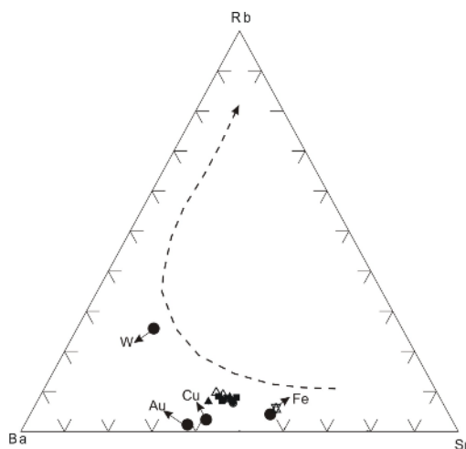
شکل ۱۰ مثلث Rb-Ba-Sr [۲۰] و میانگین نفوذی همراه با اسکارن‌های مختلف بریتیش کلمبیا [۳۱] (دوایر تو پر) به همراه نمونه‌های گرانیتوئیدی منطقه‌ی مورد بررسی (علائم مانند شکل ۵)، (پیکان خط چین راستای جدایش را نشان می‌دهد).
