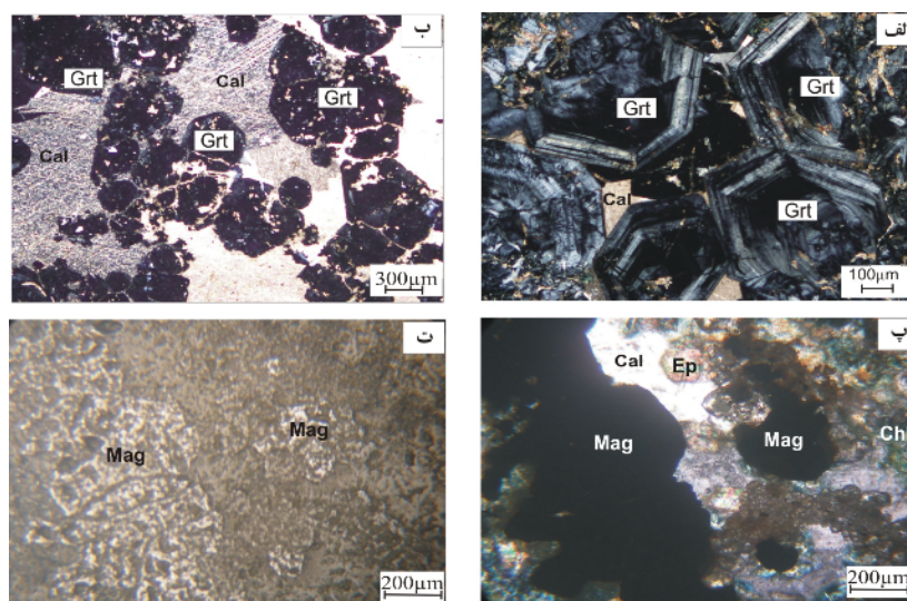
شکل ۴ (الف و ب) تصاویر میکروسکوپی از گارنت اسکارن‌های منطقه‌ی مورد بررسی (XPL)؛ (پ و ت) جانشینی مگنتیت به جای گارنت و همراهی آن با مجموعه کانی‌های کلریت و اپیدوت (هر دو تصویر یک گستره را نشان می‌دهد)؛ (پ: نور عبوری، XPL)؛ (ت: نور بازتابی، PPL)
