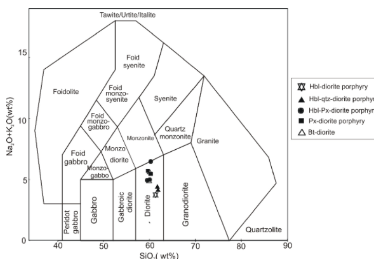
شکل ۵ نامگذاری سنگ‌های نفوذی - نیمه نفوذی بیشه با استفاده از [۱۷].
