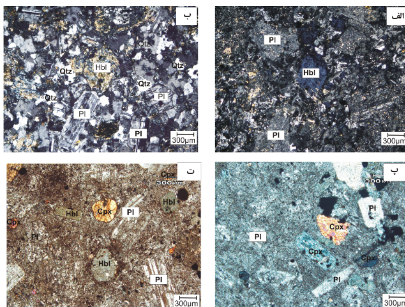
شکل ۳ تصاویر میکروسکوپی از: (الف) هورنبلند دیوریت پورفیری؛ (ب) هورنبلند کوآرتز دیوریت پورفیری؛ (پ) پیروکسن دیوریت پورفیری و (ت) هورنبلند پیروکسن دیوریت پورفیری منطقه‌ی مورد بررسی (XPL).
