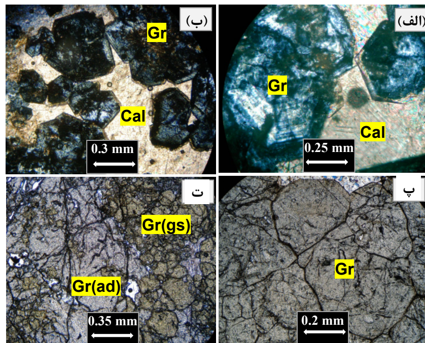
شکل ۳ رخداد گارنت در اسکارن دره‌ی زرشک؛ (الف) منطقه‌بندی نوسانی و ماکل پروانه‌ای در گارنت (XPL)؛ (ب) بلورهای گارنت ناهمسانگرد خوش وجه با منطقه‌بندی نوسانی و پروانه‌ای در زمینه‌ی کلسیت (XPL)؛ (پ) بافت موزائیکی ناشی از رشد تعادلی بلورهای خوش وجه گارنت با زوایای بین بلوری ۱۲۰ درجه (PPL)؛ (ت) درهم رشدی گارنت آندرادیتی با گارنت گراسولاری (PPL). علائم اختصاری: Gr: گارنت، Cal: کلسیت، Gr(g): گارنت گراسولاری، Gr(ad): گارنت آندرادیتی.
