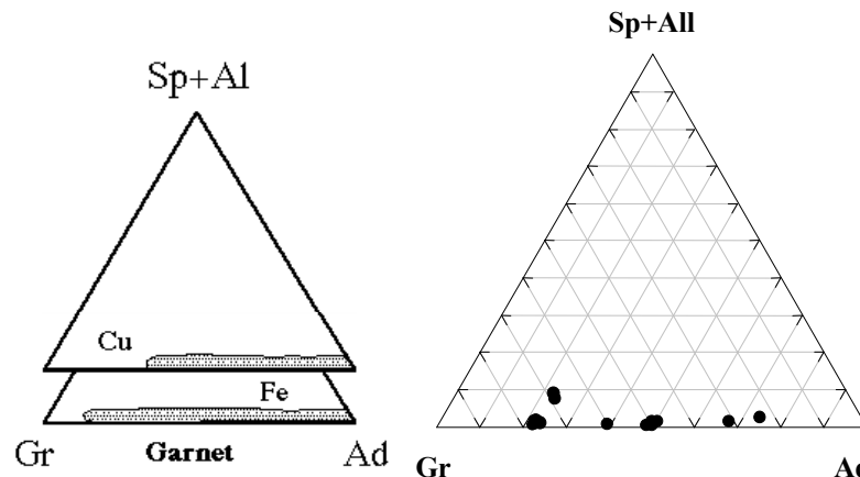
شکل ۹ نمودار توزیع ترکیب تجزیه‌های ریزکالندهی الکترونی گارنت‌های اسکارن دره‌ی زرشک و مقایسه آن‌ها با ترکیب گارنت‌های انواع نهشته-های اسکارنی [۱۱،۱۰]. علائم اختصاری: Gr: گراسولار، Ad: آندرادیت، Sp: اسپسارتین، Al: آلماندن.
