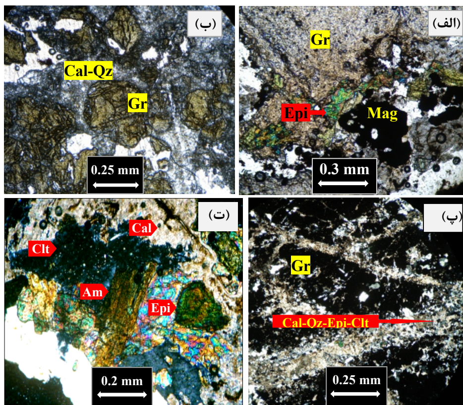
شکل ۴ (الف) تشکیل مگنتیت و اپیدوت از راه جانشینی گارنت (PPL)؛ (ب) خردشدگی و سیمانی شدن گارنت به وسیله‌ی کوارتز و کلسیت در مرحله‌ی دگرسانی قهقرایی (PPL)؛ (پ) قطع اسکارن پیشرونده با رگچه‌های اسکارن قهقرایی (XPL)؛ (ت) تشکیل کلریت از راه جانشینی اپیدوت و آمفیبول در مرحله‌ی دگرسانی پسرونده (XPL)؛ (د) علایم اختصاری: Gr: گارنت، Mag: مگنتیت، Epi: اپیدوت، Cal: کلسیت، Qz: کوارتز، Clt: کلریت، Am: آمفیبول.
