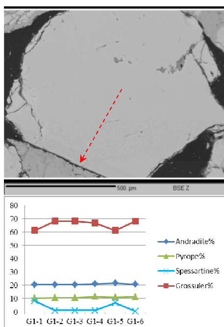
شکل ۱۱ تصویر BSE کانی گارنت و نمودار درصد تغییرات نوع گارنت در راستای پیمایش (مرکز به حاشیه) ریزکاوته‌ی الکترونی (داده‌های پیمایش ۱ در جدول ۲).
