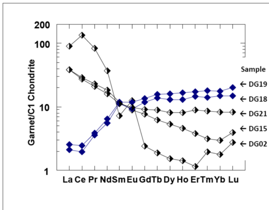
شکل ۷ الگوی رفتاری عناصر کمیاب خاکی در گارنت‌های اسکارن دره‌ی زرشک. علائم اختصاری: DG02، DG15 و DG21 گارنت‌های با ترکیب آندرادیتی، DG18 و DG19 گارنت‌های با ترکیب گراسولاری.
