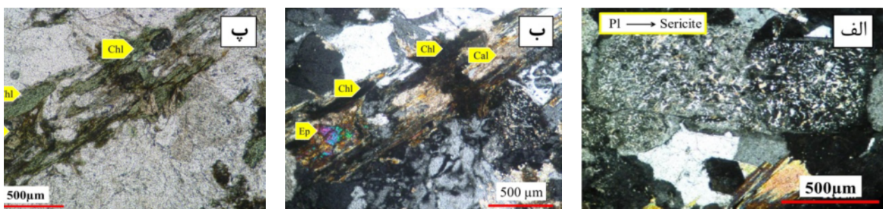
شکل ۲ الف: دگرسانی کامل پلاژیوکلاز به سریسیت در گرانودیوریت‌های منطقه‌ی پناهکوه - ب و پ دگرسانی پلاژیوکلاز به کانی‌های کلریت، اپیدوت، اسفن و کلسیت در نتیجه‌ی دگرسانی پروپیلیتی (ب: نیکل عمود ج: نیکل موازی).
