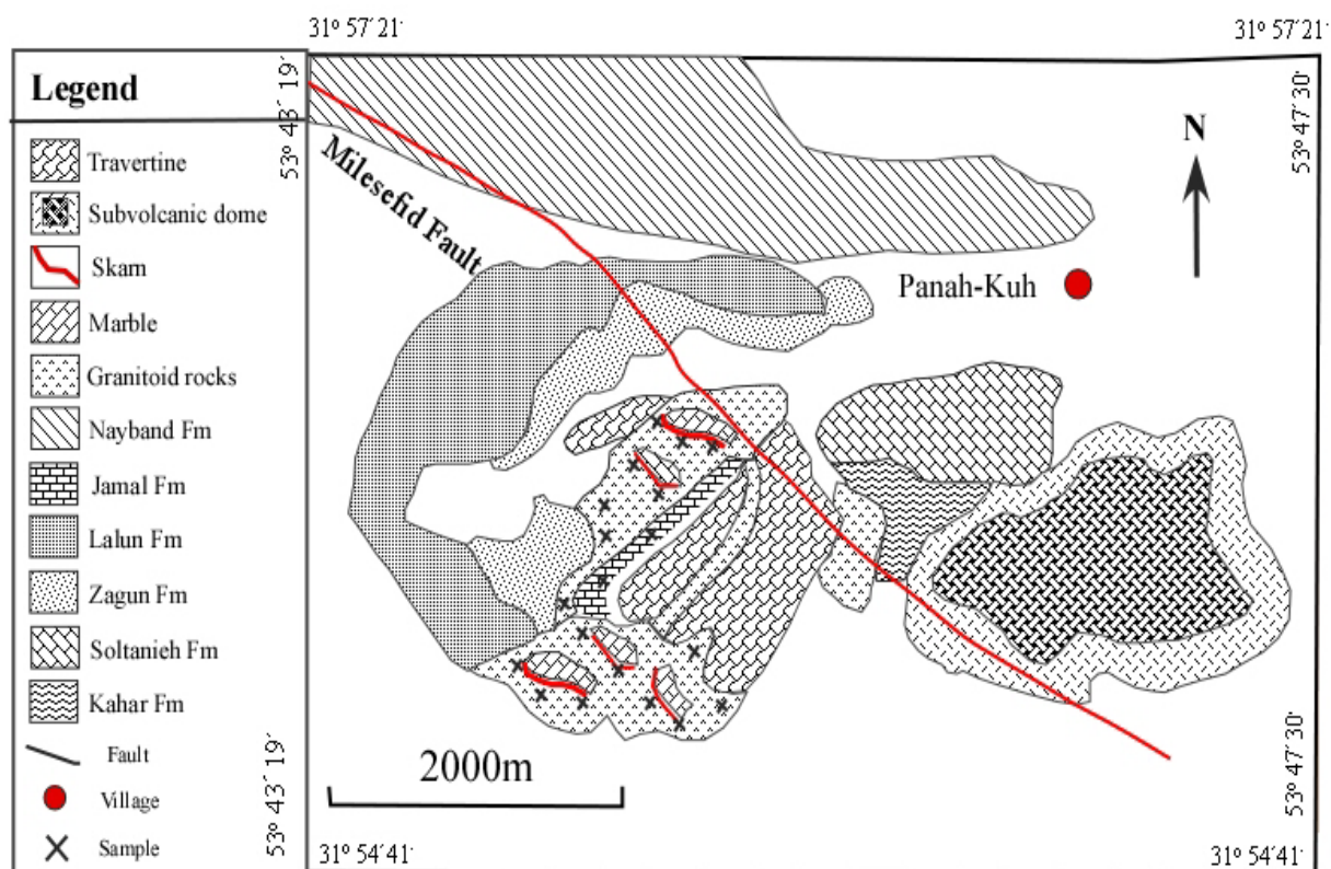
شکل ۱ نقشه‌ی زمین‌شناسی منطقه پناهکوه واقع در غرب استان یزد بر اساس مطالعات صحرایی و استفاده از عکس‌های هوایی (اقتباس از نقشه زمین‌شناسی ۱:۱۰۰۰۰۰ خضرا باد با تغییرات).
