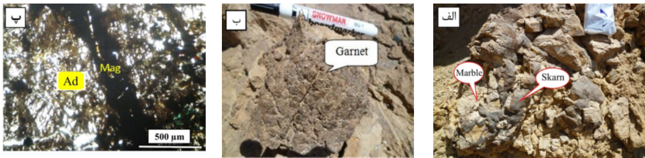
شکل ۴ الف: برشی شدن مرمرها و اسکارن‌های همراه آن ب: گارنت اسکارن با بیش از ۹۰ درصد گارنت پ: گارنت‌های همسانگرد بی‌شکل با شکستگی‌های فراوان که با اکسیدهای آهن پر می‌شود.
