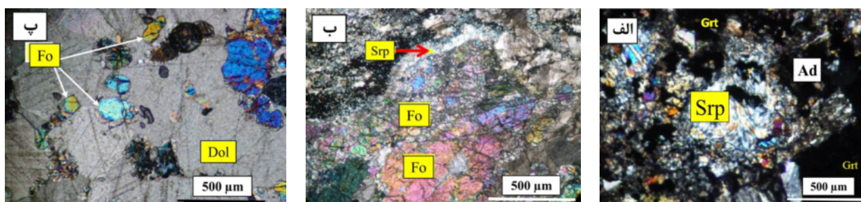
شکل ۷ الف جانشینی کامل اولیوین با سرپانتین و تشکیل شبريخت حاصل از آن ب: سرپانتینی شدن اولیوین و تشکیل بافت شبکه‌ای حاصل از آن در اسکارن منیزی. پ: درشت بلورهای اولیوین سالم با پیرامون گرد شده (Resorbed) در اسکارن منیزی.
