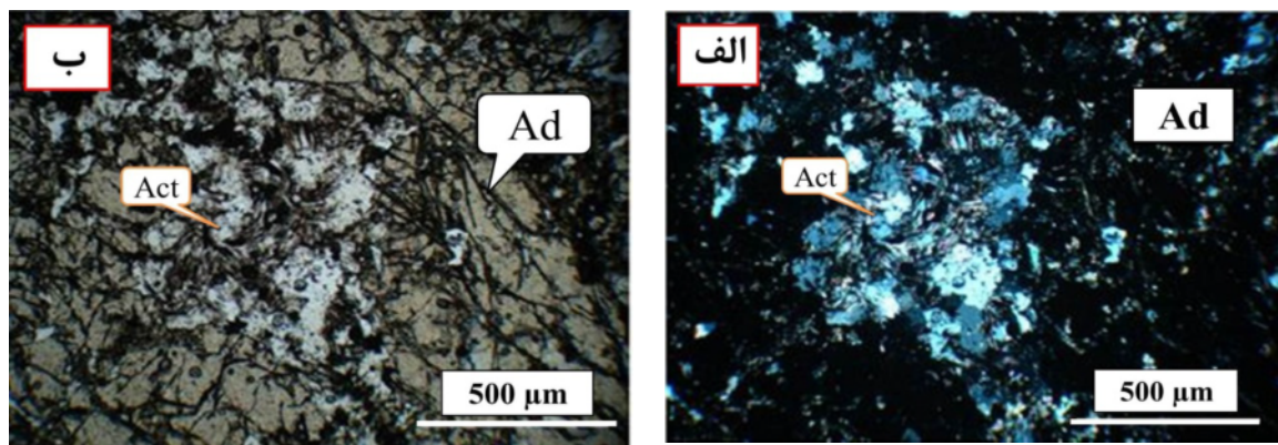
شکل ۱۰ قرار گرفتن اکتینولیت به صورت مستقل و در همراهی با کوارتز در فضای بین آندرادیته‌ها (الف: نیکل عمود ب: نیکل موازی).
