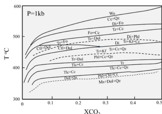
شکل ۱۳ نمودار روابط فازي T- X_{CO_2} در سامانه Al-K-Ca-Mg-Si-H-C-O [۱۲].
