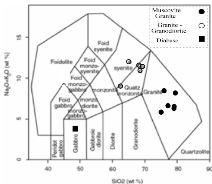
شکل ۶ رده بندی سنگ‌های مورد بررسی بر اساس [۲۷].
