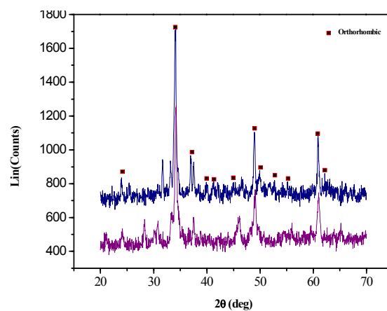
شکل ۳ الگوهای پراش پرتو X نمونه‌های تهیه شده به روش الف) واکنش حالت جامد و ب) سل-ژل پس از برشتن در دمای 800^\circ\text{C} .
