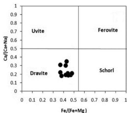
شکل ۴ موقعیت کانی شناختی تورمالین بر اساس موقعیت X و Y با ترکیب دراویت [۱۴].
