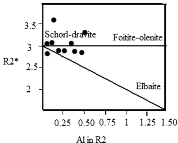
شکل ۶ موقعیت کانی شناختی تورمالین در نمودار R2* برابر Al in R2 [۵].
