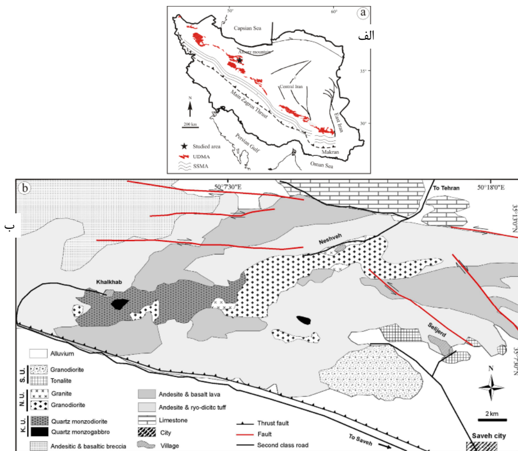
شکل ۱ نقشه‌ی زمین شناسی منطقه که از نقشه زمین شناسی ۱:۱۰۰۰۰۰ ساوه [۱۱] که توسط [۱۵، ۱۴] تصحیح گردیده، اقتباس شده است.
