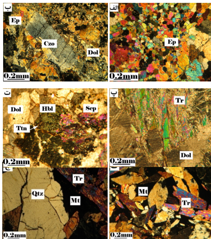
شکل ۱۱ تصاویر میکروسکوپی نمونه‌های اسکارنی منطقه در نور XPL. (الف) اسکارن اپیدوتیتی. (ب) اسکارن اپیدوت و کلینوزوئیزیت‌دار (پ) اسکارن ترمولیت‌دار (ت) اسکارن ترمولیت و اسکاپولیت‌دار (ث) اسکارن ترمولیت و مگنتیت‌دار (ج) اسکارن ترمولیت، مگنتیت و کوارتزدار. Ep: اپیدوت، Czo: کلینوزوئیزیت، Dol: دولومیت، Tr: ترمولیت، Sep: اسکاپولیت، Ttn: تیتانیت، Mt: مگنتیت.
