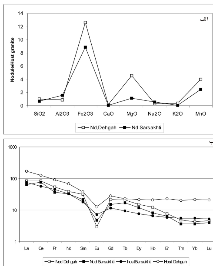
شکل ۳ الف- ترکیب شیمیایی عناصر اصلی گرهمهای تورمالین عادی شده به سنگ میزبان آنها ب- نمودار عناصر نادر خاکی که نسبت به کاندیت [۲۱] نرمال شده اند.
