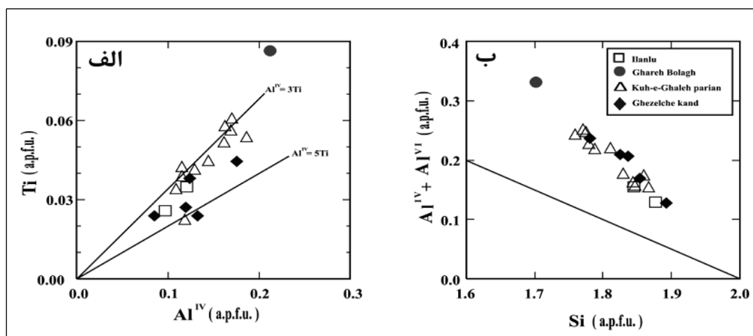
شکل ۴ الف) ترکیب شیمیایی کلینوپیروکسن‌های منطقه‌ی شمال شرق قروه روی نمودار تغییرات Al^{IV} -Ti، ب) ترکیب شیمیایی کلینوپیروکسن‌های منطقه‌ی شمال شرق قروه روی نمودار Al-Si.
