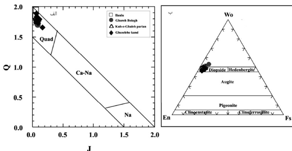
شکل ۳ الف) همه‌ی پیروکسن‌های منطقه‌ی شمال شرق قروه در نمودار Q-J [۱۵]، در قلمرو پیروکسن‌های Ca - Fe - Mg (Quad) قرار می‌گیرند ( Q = Ca + Mg + Fe^{2+} و J = 2Na ). ب) ترکیب شیمیایی کلینوپیروکسن‌های منطقه‌ی شمال شرق قروه روی نمودار مثلی Wo - En - Fs [۱۵] در گستره‌ی دیوپسید قرار دارند.
