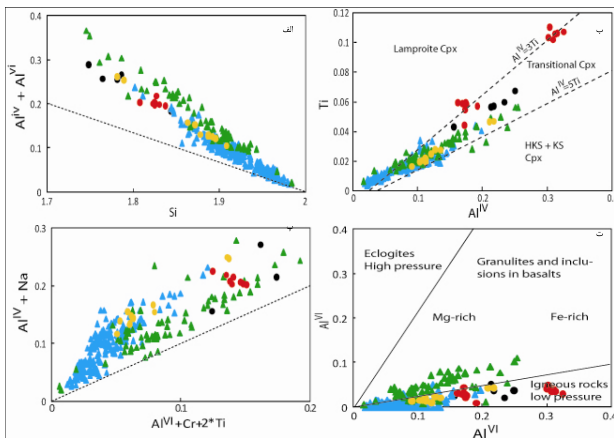
شکل ۷ (الف) نمودار توزیع \text{Al}^{\text{IV}} نسبت به Si [۲۱]، (ب) نمودار Ti نسبت به \text{Al}^{\text{IV}} [۱۶، ۲۶]، (پ) نمودار \text{Al}^{\text{IV}} + \text{Na} نسبت به \text{Al}^{\text{VI}} + \text{Cr} + 2 \cdot \text{Ti} [۲۱]، (ت) نمودار توزیع آلومینیوم در موقعیت چهاروجهی و هشت وجهی [۲۷]. علایم همانند شکل ۴ انتخاب شدند.
