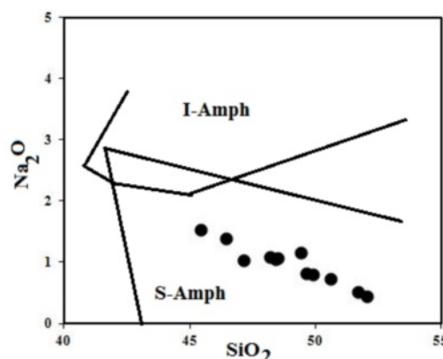
شکل ۷ نمودار رده‌بندی تکتونوماگمایی آمفیبول‌های گرانیتوئید بزمان.
