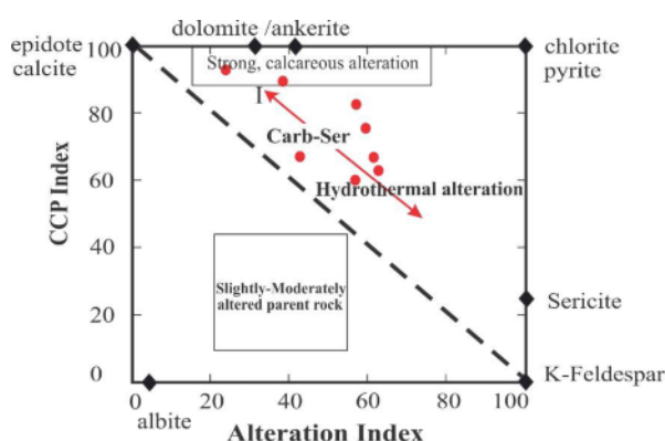
شکل ۷ نمودار جعبه‌ای دگرسانی [شاخص دگرسانی ایشیکاوا ( AI ) نسبت به شاخص دگرسانی کلریت-کربنات-پیریت ( CCPI )] برای داده‌های تجزیه‌ی شیمیایی منطقه‌ی مورد بررسی. روند اصلی دگرسانی با روند I (دگرسانی سیریسیتی-کربناته) نشان داده شده است.
