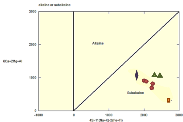
شکل ۱۲ موقعیت سنگ‌های گرانیتوئیدی کوهریگی در قلمرو شبه-قلیایی [۱۰].
