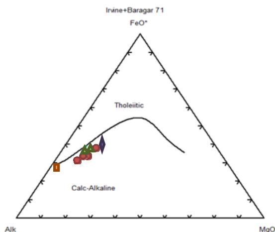
شکل ۱۳ نمودار AFM، سنگ‌های مورد مطالعه در محدوده کالک آلکالین قرار می‌گیرند [۱۱].
