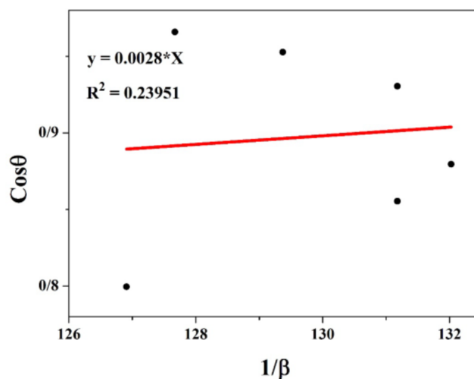
شکل ۲ محاسبه اندازه بلورک نمونه بازپخت شده در دمای 400^{\circ}C به روش شرر.
