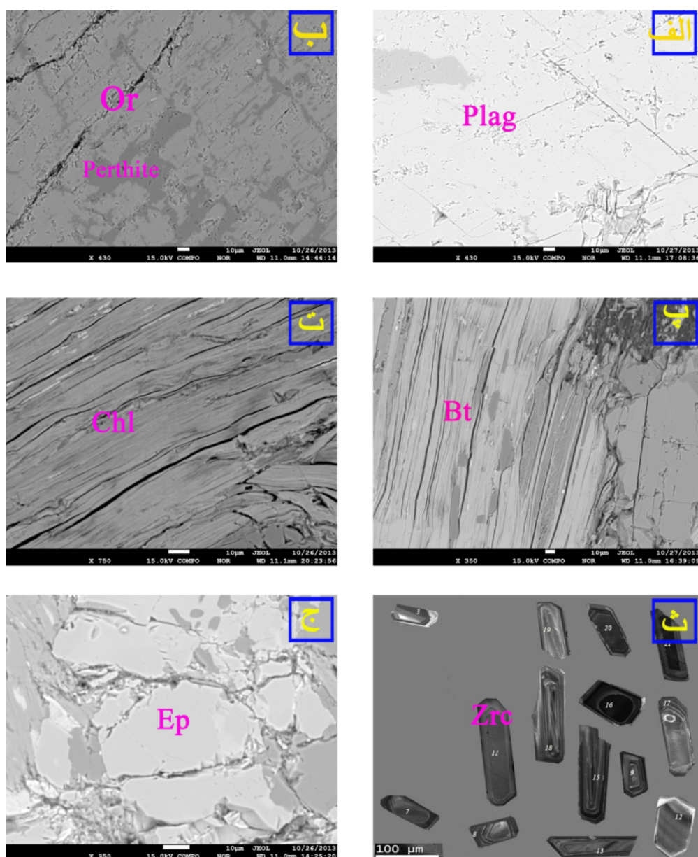
شکل ۳ الف تا ج- تصاویر میکروسکوپ الکترونی (BSE)(Back-Scattered Electrons) تهیه شده به ترتیب از کانی‌های ارتوز، پلاژیوکلاز، کلریت، بیوتیت و اپیدوت در گرانیته‌ها. ث- تصاویر رخشانی کاندی از دانه‌های زیرکن جدا شده از گرانیته‌ها.
