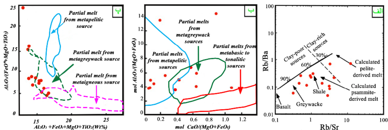
شکل ۸ الف، ب و ب- موقعیت نمونه‌های مورد بررسی به ترتیب روی نمودارهای تغییرات \text{Rb}/\text{Ba} نسبت به \text{Rb}/\text{Sr} [۲۶]، \text{mol Al}_2\text{O}_3/(\text{MgO}+\text{FeO}) در برابر \text{mol CaO}/(\text{MgO}+\text{FeO}) [۲۷] و \text{Al}_2\text{O}_3/(\text{FeO}+\text{MgO}+\text{TiO}_2) نسبت به \text{Al}_2\text{O}_3+\text{FeO}+\text{MgO}+\text{TiO}_2 (Wt%) [۲۵]. نمونه‌ها بیشتر در گستره‌های با سنگ‌خاستگاه متاگرایوکی و متاپلیت فقیر از رس قرار می‌گیرند.
