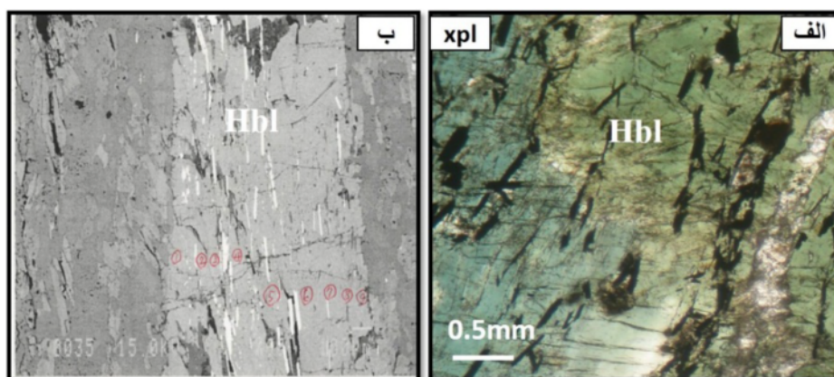
شکل ۸ (الف) تصویر میکروسکوپی هورنبلند (Hbl) سبز-آبی گلوگاه در نمونه‌ی B3، (ب) تصویر BSE هورنبلند آنالیز شده در نمونه‌ی B3 با مقیاس 100 \mu m.
