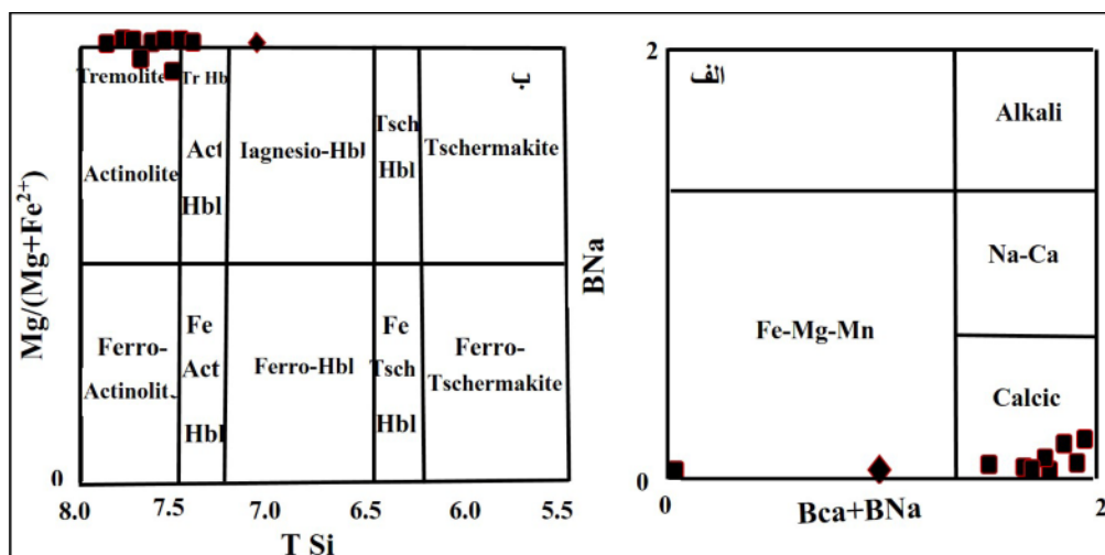
شکل ۶ نمودارهای رده بندی آمفیبول‌ها بر پایه ترکیب شیمیایی آن‌ها [۲۱]، الف) موقعیت آمفیبول‌های موجود در شبه‌پریدوتیت‌های همبافت دگرگون ده‌سلم، بیشتر نمونه‌ها در گستره‌ی کلسیک قرار دارند؛ ب) موقعیت آمفیبول‌های کلسیک مورد بررسی، نمونه‌ها در گستره‌ی ترمولیت، هورنبلند ترمولیتی و هورنبلند منیزیم‌دار قرار دارند. (■ = متاپریدوتیت اسپینل‌دار، ◆ = متاپریدوتیت تالک‌دار).
