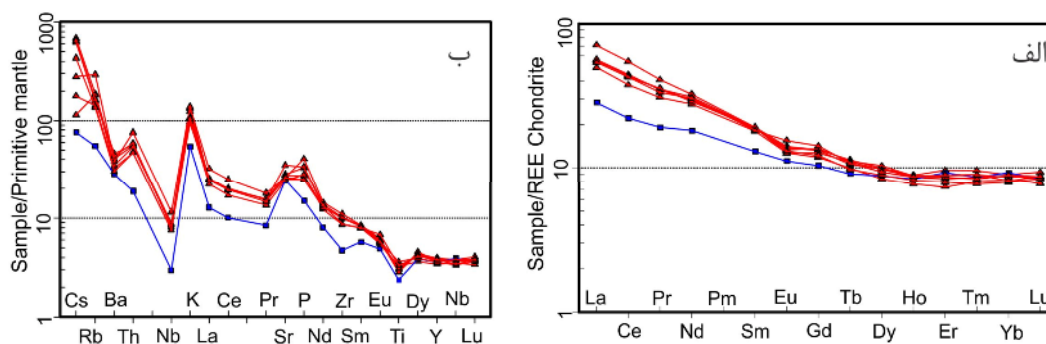
شکل ۱۳ نمودار عناصر خاکی نادر بهنجار شده به کاندزیت (الف) و عناصر فرعی و برخی خاکی نادر بهنجار شده به گوشته اولیه (ب) برای نمونه‌های سنگ آتشفشانی کانسار چشمه گز. مقادیر اولیه کاندزیت از [۱۰] و گوشته اولیه از [۱۵].
