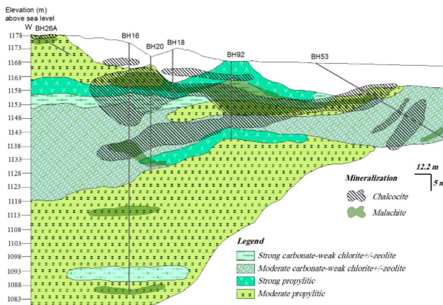
شکل ۶ مقطع دگرسانی - کانی‌سازی زیرسطحی غرب کانسار چشمه گز (نسیم).
